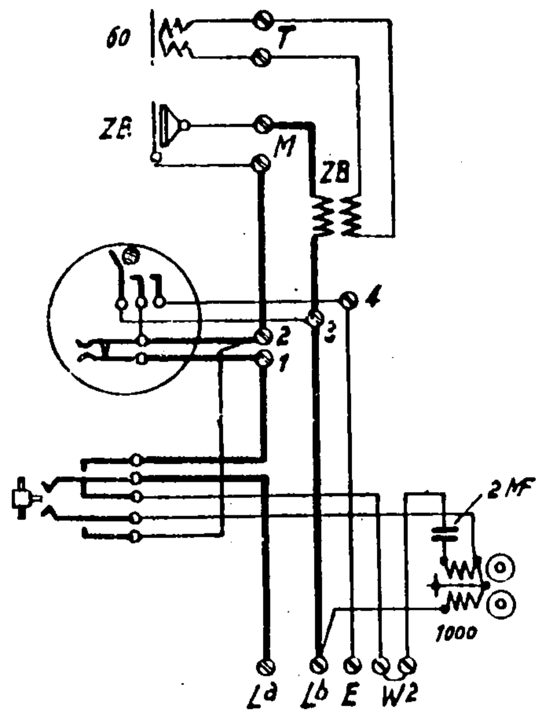
Abb. 36. ZB-App. ohne Rückfrage. AS-300 ohne Wählscheibe. AS-300a mit Wählscheibe.
