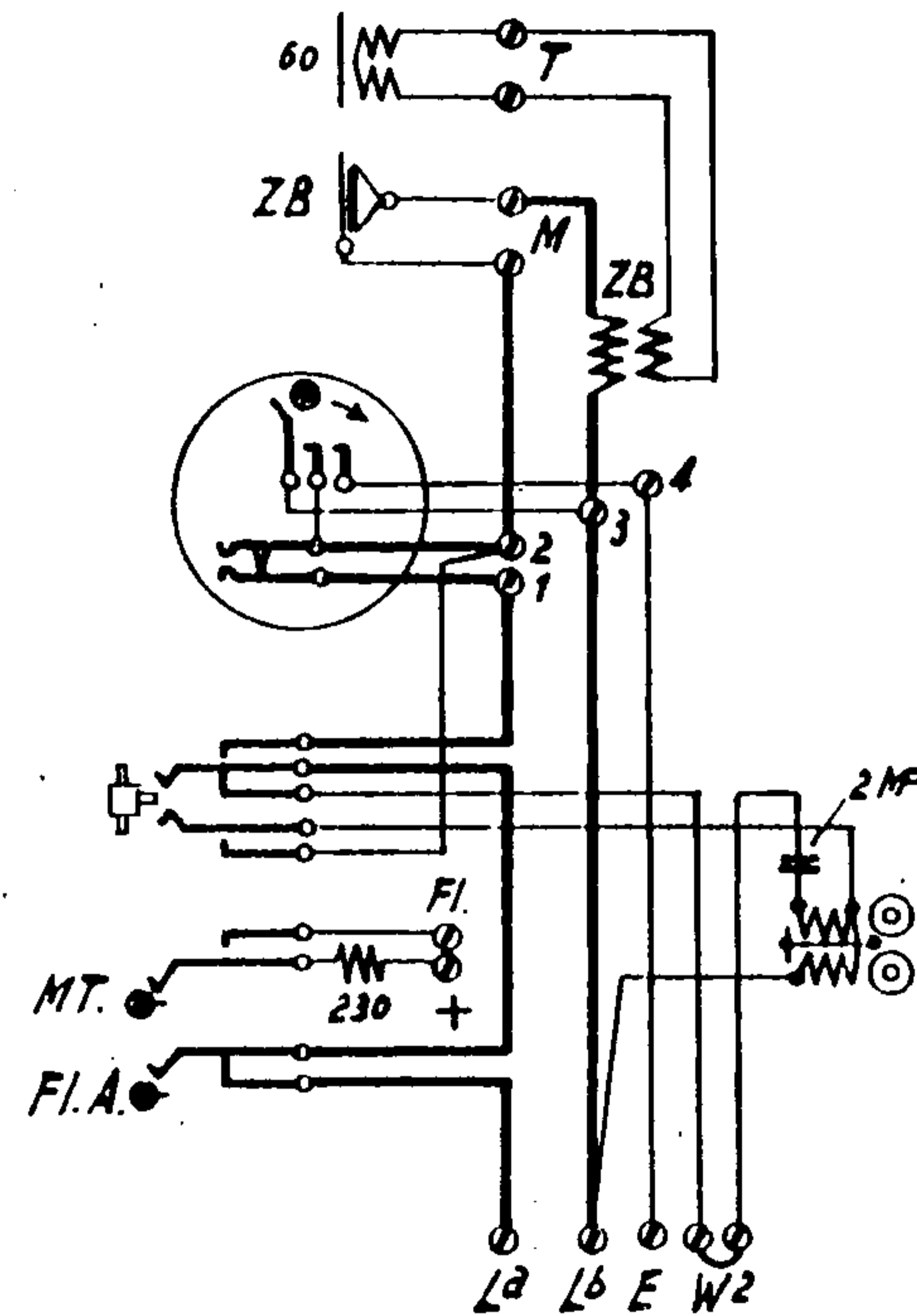
Abb. 37. ZB-App. ohne Rückfrage m. Melde- u. Flackertaste. AS-300/10 ohne Wählscheibe. AS-300/10a mit Wählscheibe.
